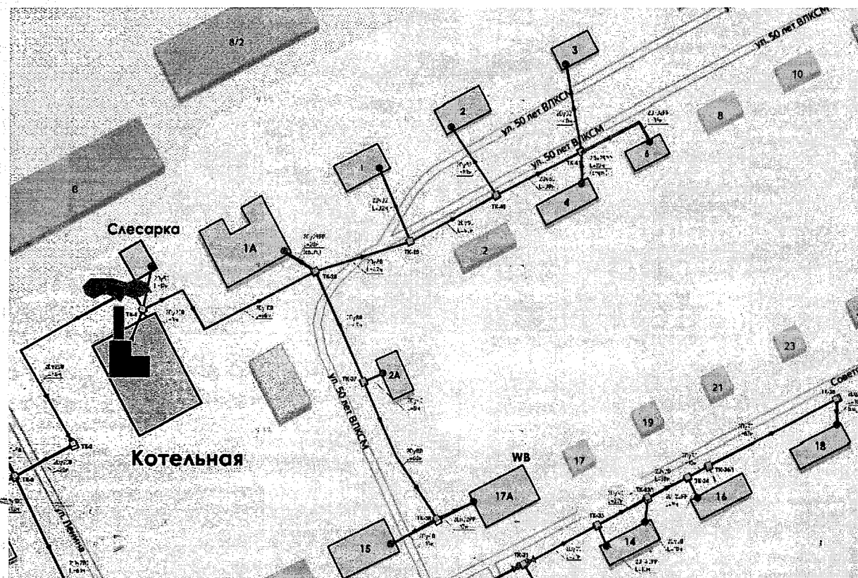
Рисунок 7.4.3. vk Визуализация отключения участка тепловой сети
