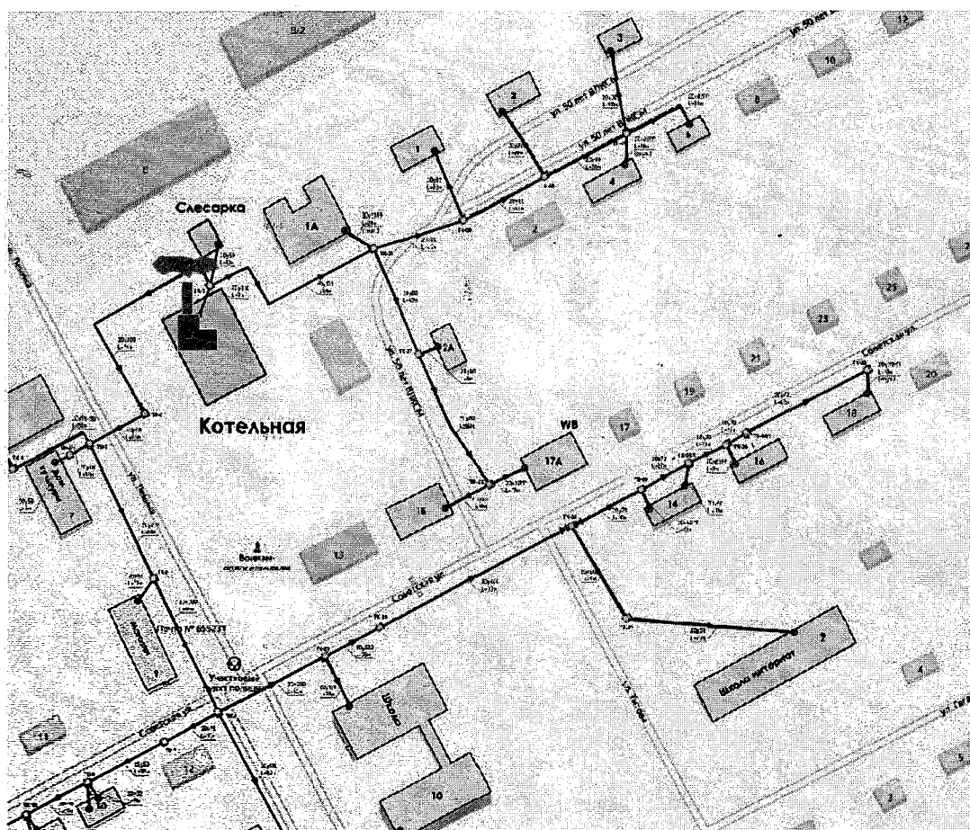
Рисунок 7.4.2. Визуализация отключения участка тепловой сети
